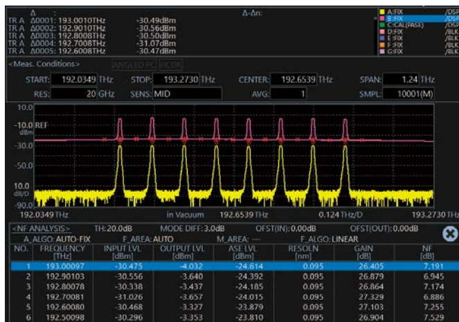
AQ6370E测量波形示例
