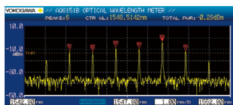
光谱显示示例
