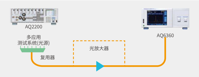
光放大器测试的典型实验设置
