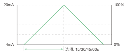
线性扫描源示例
