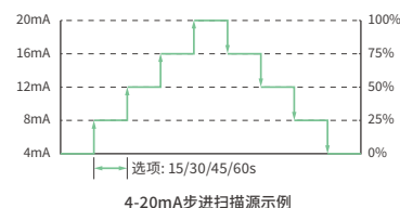
4-20mA步进扫描源示例
