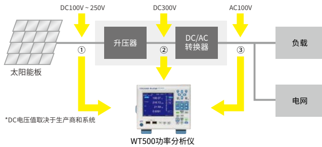
光伏功率调节器的概要图
