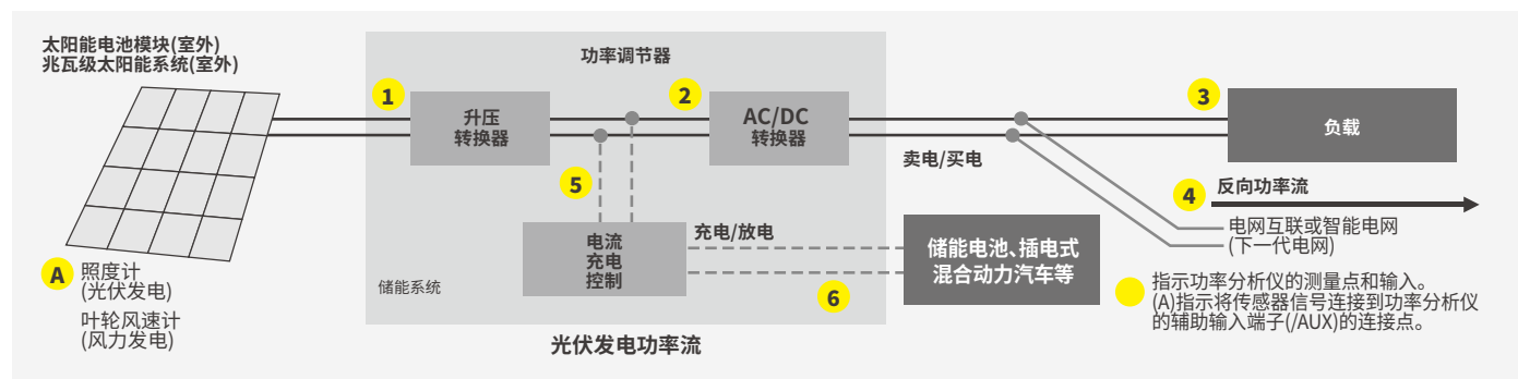
MPPT控制中的典型电压、电流和功率测量
