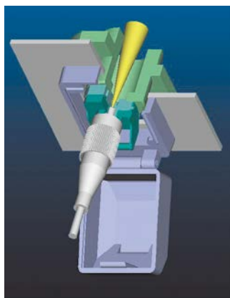
光输入结构
