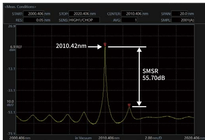
2010nm DFB-LD的测量示例
