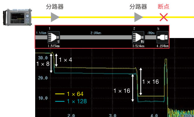
128/64端口分路器测量示例
