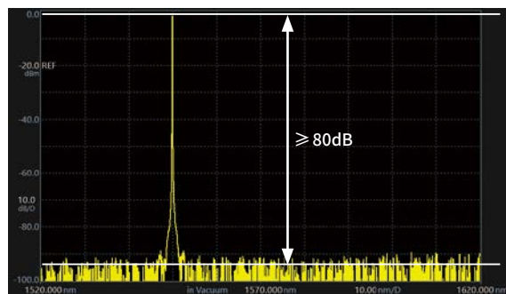
杂散光抑制性能
