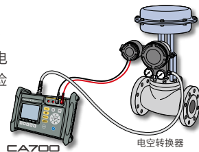
电空转换器
