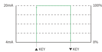
4-20mA范围检查示例
