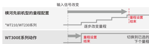
量程跳转(配置)功能运行图
