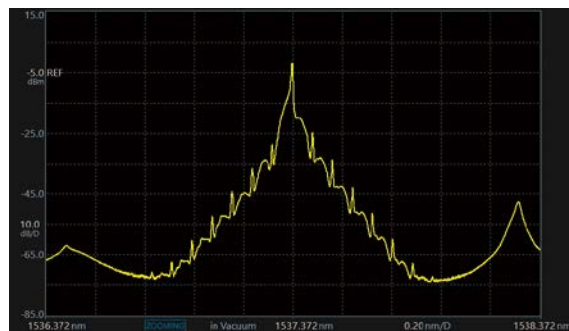
10G光收发器的调制光谱
