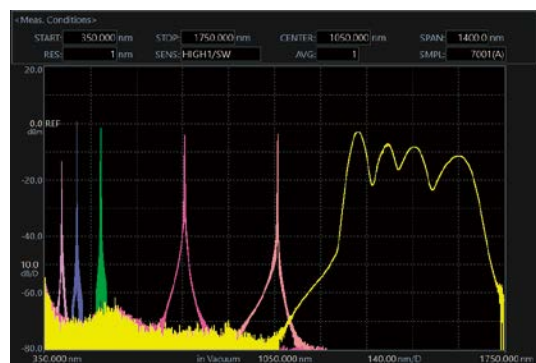
激光器和宽带光源的测量示例 (5 FP-LD和 SLD光源)
