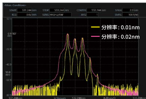
高分辨率机型的可见激光测量示例
