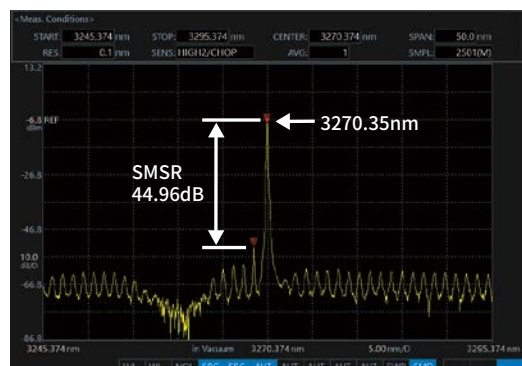
3270nm DFB-LD的测量示例(分辨率: 0.1nm, 跨度: 50nm)
