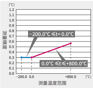
[示例]测量精度: Pt100 (3851)
