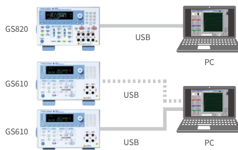
系统构成图
