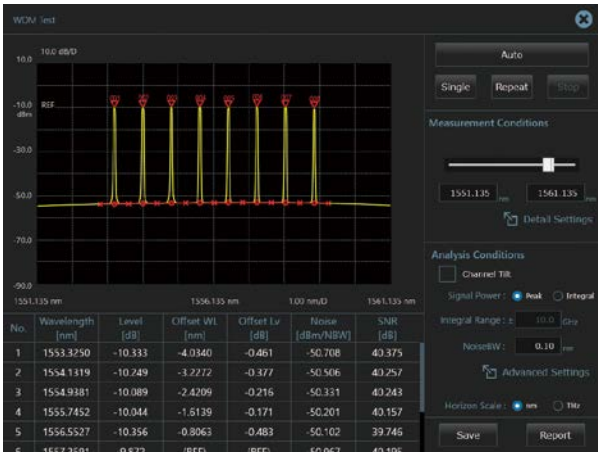
WDM测试应用
