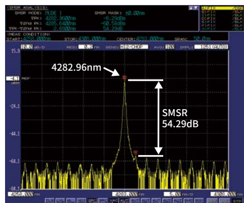
4.3μm DFB激光器的测量示例 (分辨率: 0.2nm, 跨度: 50nm)
