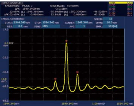
可以快速、准确地测量激光边模抑制比(SMSR)。
