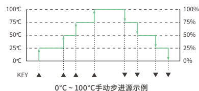
0°C ~ 100°C手动步进源示例
