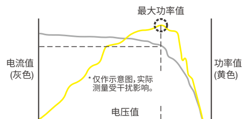
MPPT控制中的典型电压、电流和功率测量
